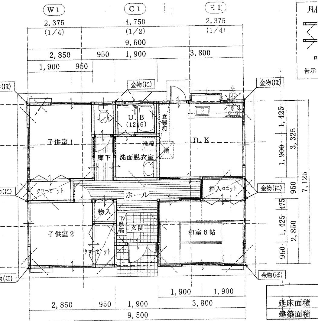
平面図 S=1/100
