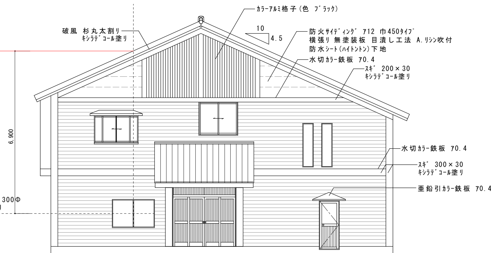
東立面図 S=1/100
