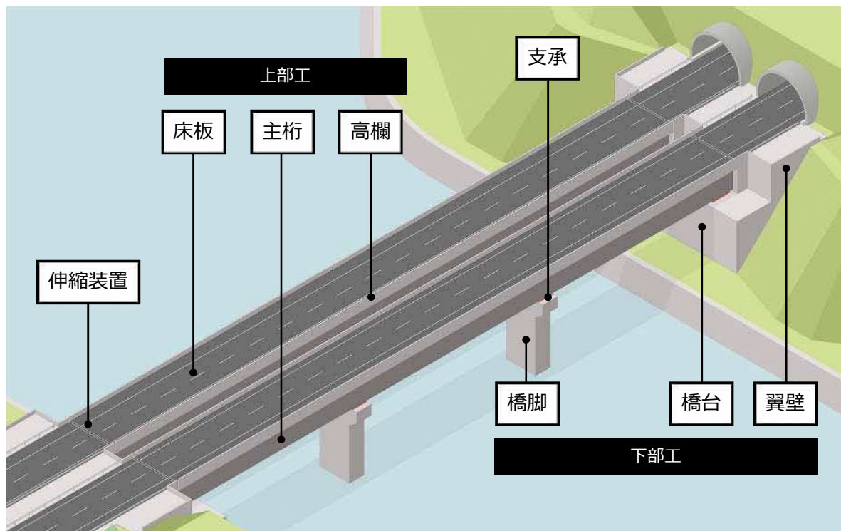
図 2 橋梁を構成する部材
