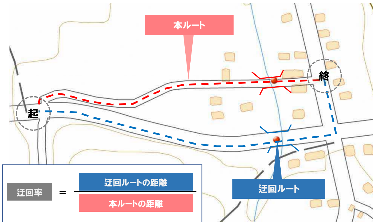
図 20 迂回率の計算方法
