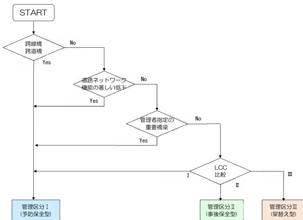
図 15 橋梁ごとの維持管理方針の最適化
