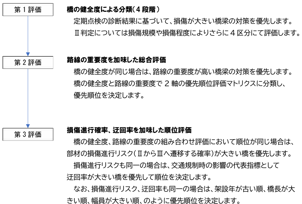
図 17 優先順位評価の流れ
