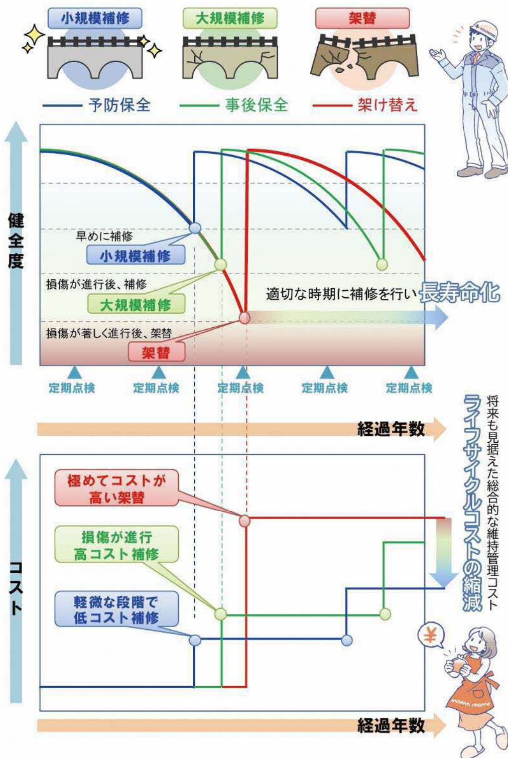
図 11 予防保全型管理手法による長寿命化とコスト縮減イメージ
